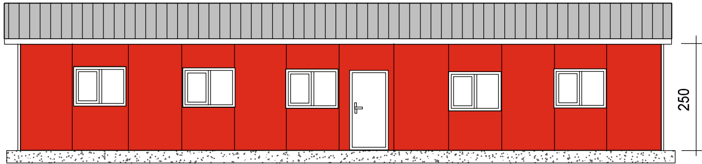
ÖN GÖRÜNÜS FRONT VIEW
