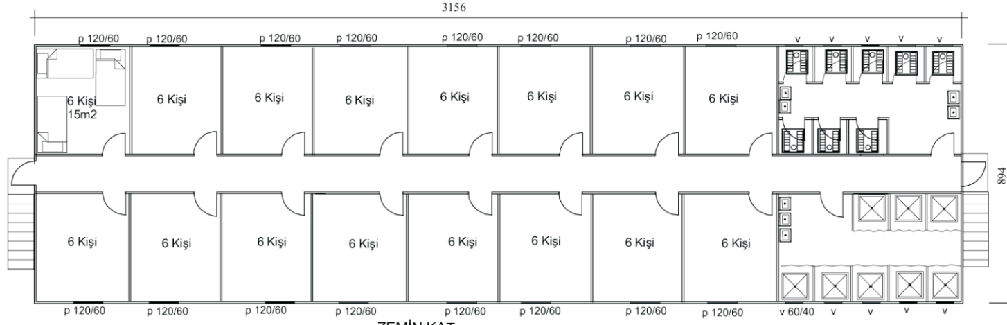
ZEMİN KAT
